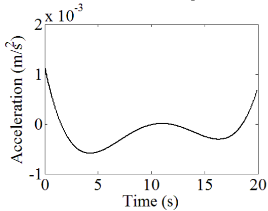
a. Q=100ml/min
