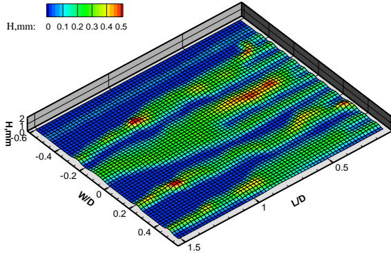
e. 100ml/min, U_\infty = 20\text{m/s}
