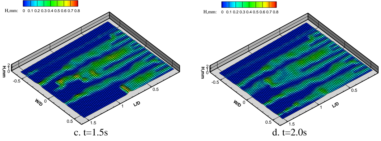
D. U_{\infty} = 20m/s, Q=100ml/min
